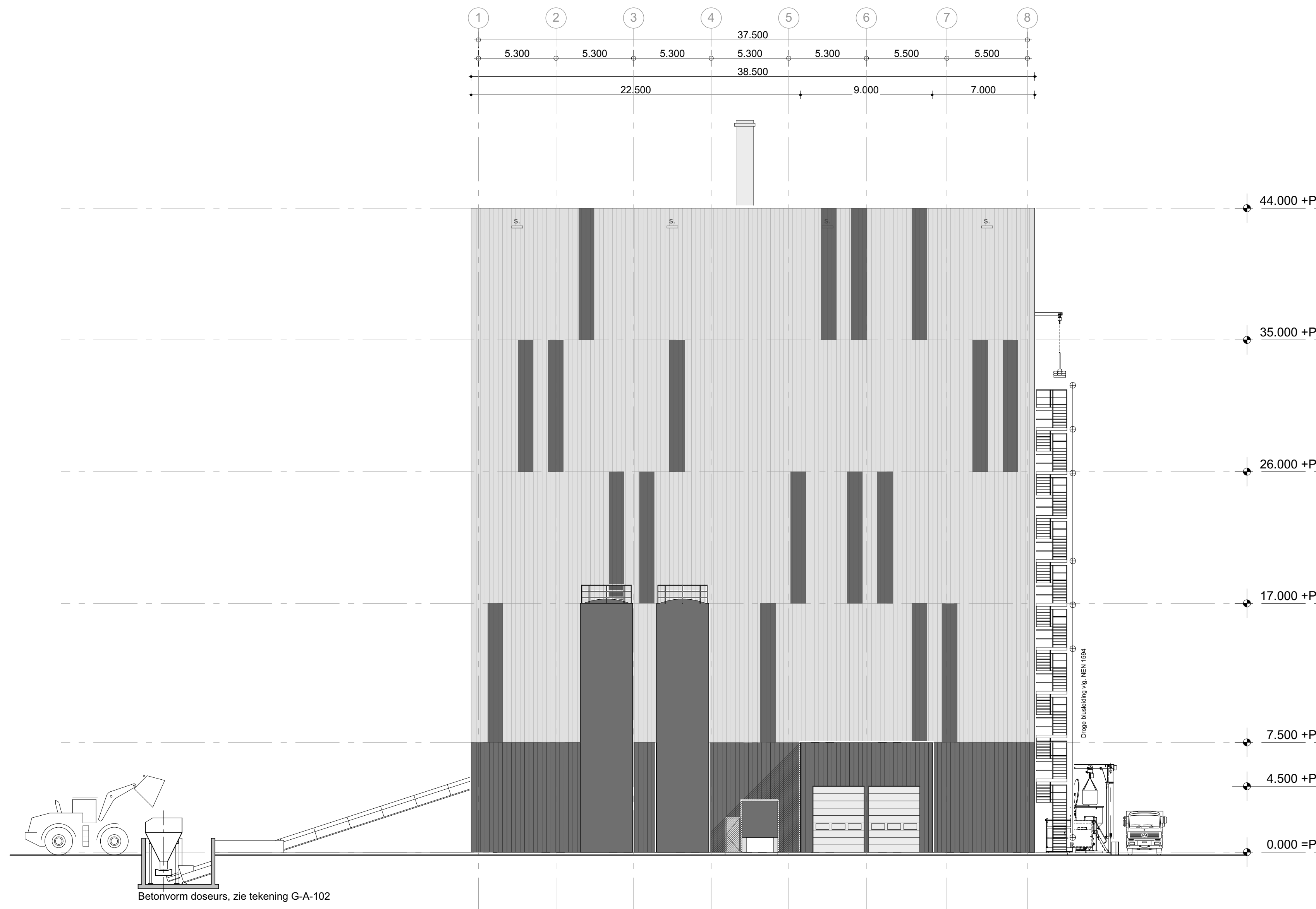
Aanzicht NOORD
