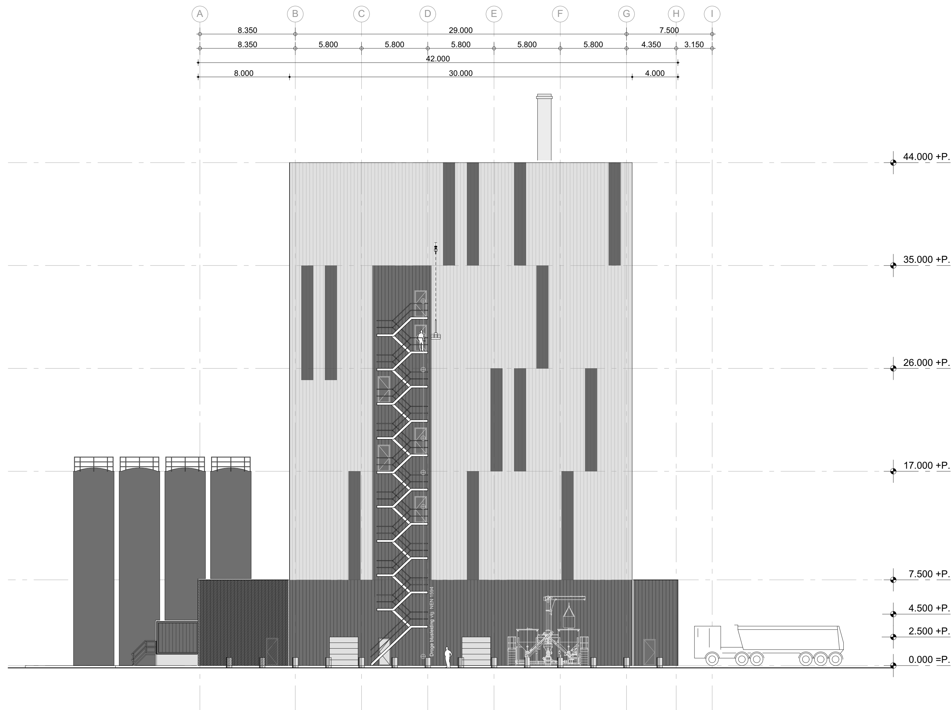
Aanzicht WEST
